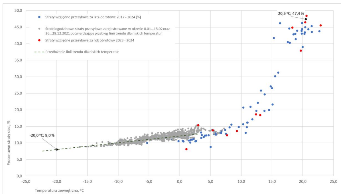
Rysunek 2 Procentowe straty sieci w sezonach 2016 - 2024
